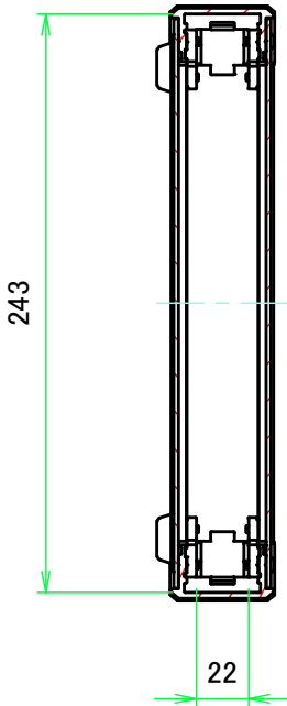
A-A ( 1 : 3.5 )
