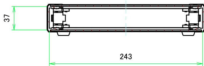
B-B ( 1 : 3.5 )
