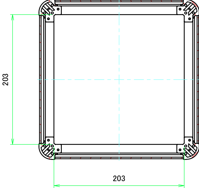
C-C ( 1 : 3.5 )
